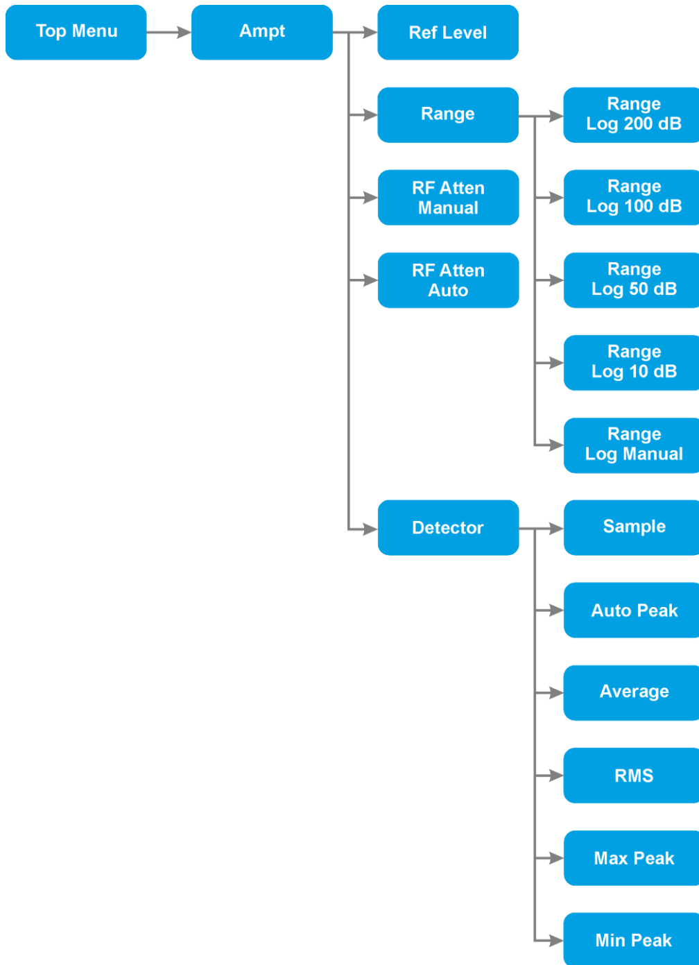
Рис. 9. Структура подменю Ampt
