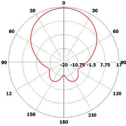
Горизонтальная плоскость
