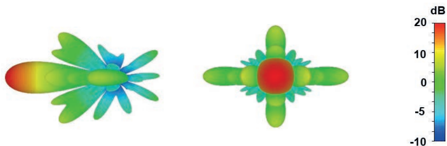
Вертикальная плоскость
