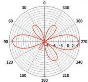
1,4 ГГц
