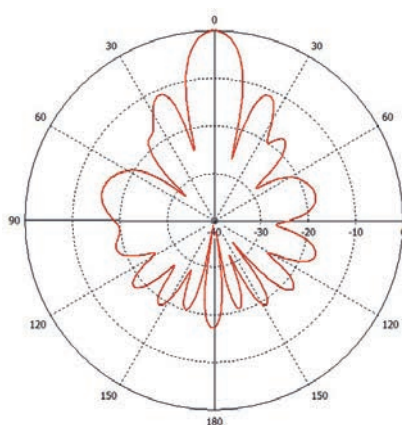
Вертикальная плоскость
