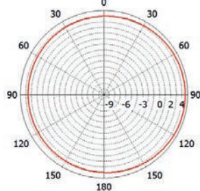
1,4 ГГц
