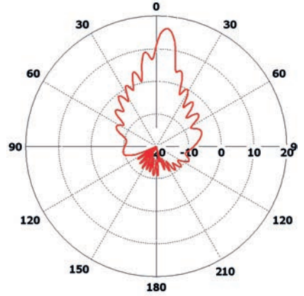
Вертикальная плоскость
