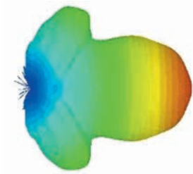
90 ГГц
