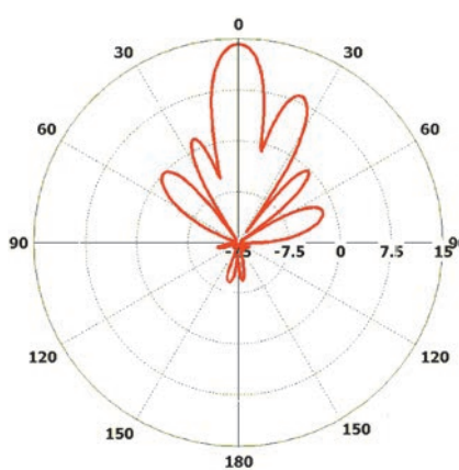
Вертикальная плоскость
