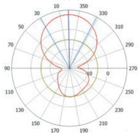
1 ГГц
