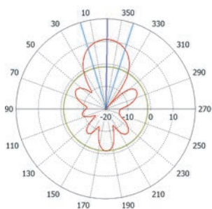
2,0 ГГц
