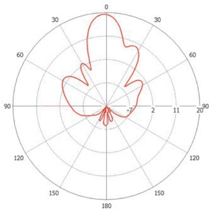
Горизонтальная плоскость
