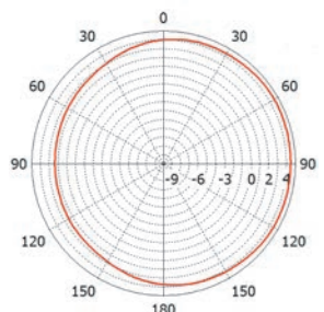
2,3 ГГц
