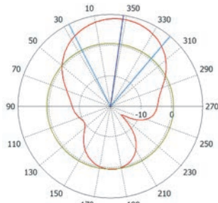
1,5 ГГц
