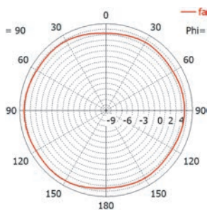
2.7 ГГц
