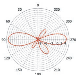
2.7 ГГц
