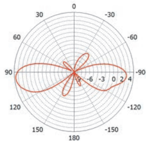
Вертикальная плоскость
