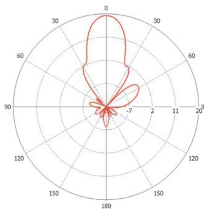
Вертикальная плоскость
