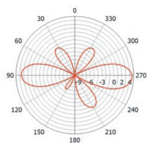
1,4 ГГц
